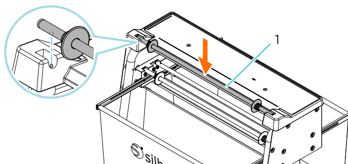
1. Barra per rotolo flangiata
